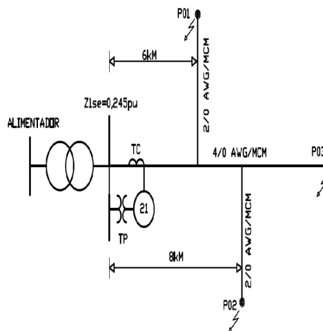
Figura 5. Exemplo de Sistema de distribuição.
