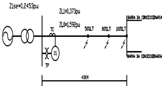
Figura 3. Exemplo de Sistema de Transmissão. Fonte: Próprio Autor.
