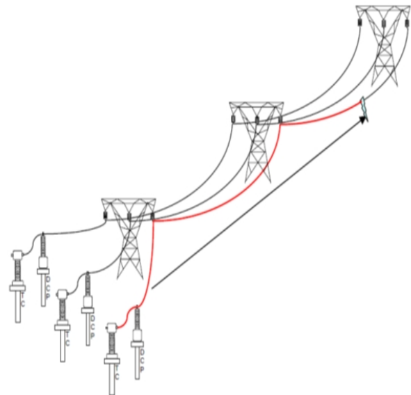
Figura 1. Impedância ser medida para uma falta fase-terra na fase A Fonte: LIMA (2006) 12 .
