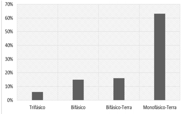
Figura 2. Ocorrências de curto-circuito. Fonte: KINDERMANN (1997) 10
